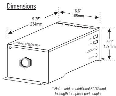
75W Halogen Luminaire
